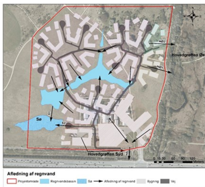
Figur 1 Planlagt aflledning af regnvand til eksisterende sø og grøfterne mod syd og øst.
